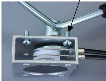
ボルトの良い取付け方
