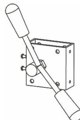
ブレーキ ON 状態
