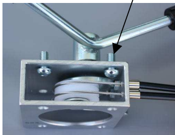
ボルトの良い取付け方
