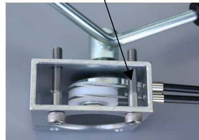
ボルトの悪い取付け方（ワイヤーにあたる）
